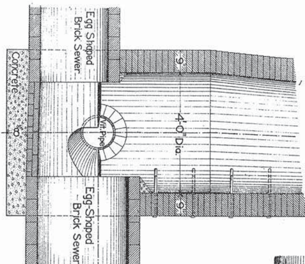
SECTION C-D
