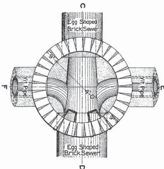
PLAN A-B
